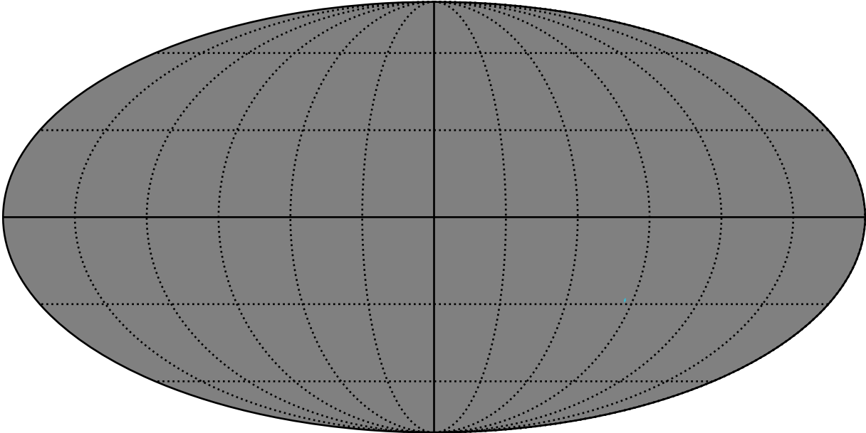
smc_lmc_v3.3_10yrs : GalplaneFootprintMetric_globular_clusters_map_Tau_20_0
