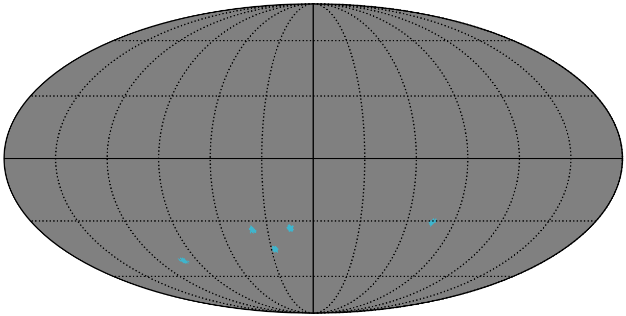
smc_lmc_v3.3_10yrs : GalplaneFootprintMetric_clementini_stellarpops_map_Tau_2_0
