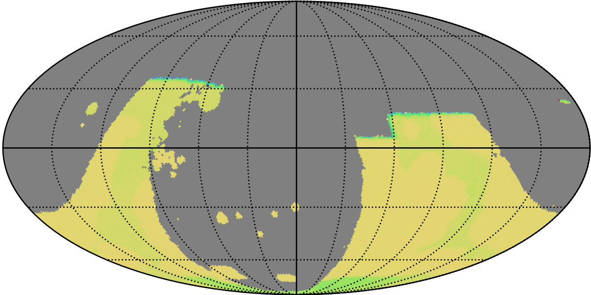
smc_lmc_v3.3_10yrs : GalPlaneVisitIntervalsTimescales_combined_map_Tau_46_5
