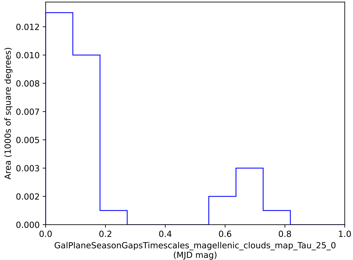
smc_lmc_v3.3_10yrs : GalPlaneSeasonGapsTimescales_magellenic_clouds_map_Tau_25_0
