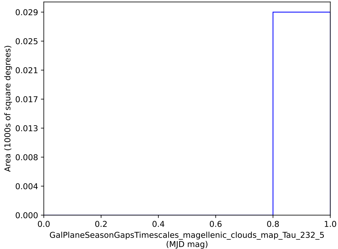
smc_lmc_v3.3_10yrs : GalPlaneSeasonGapsTimescales_magellanic_clouds_map_Tau_232_5
