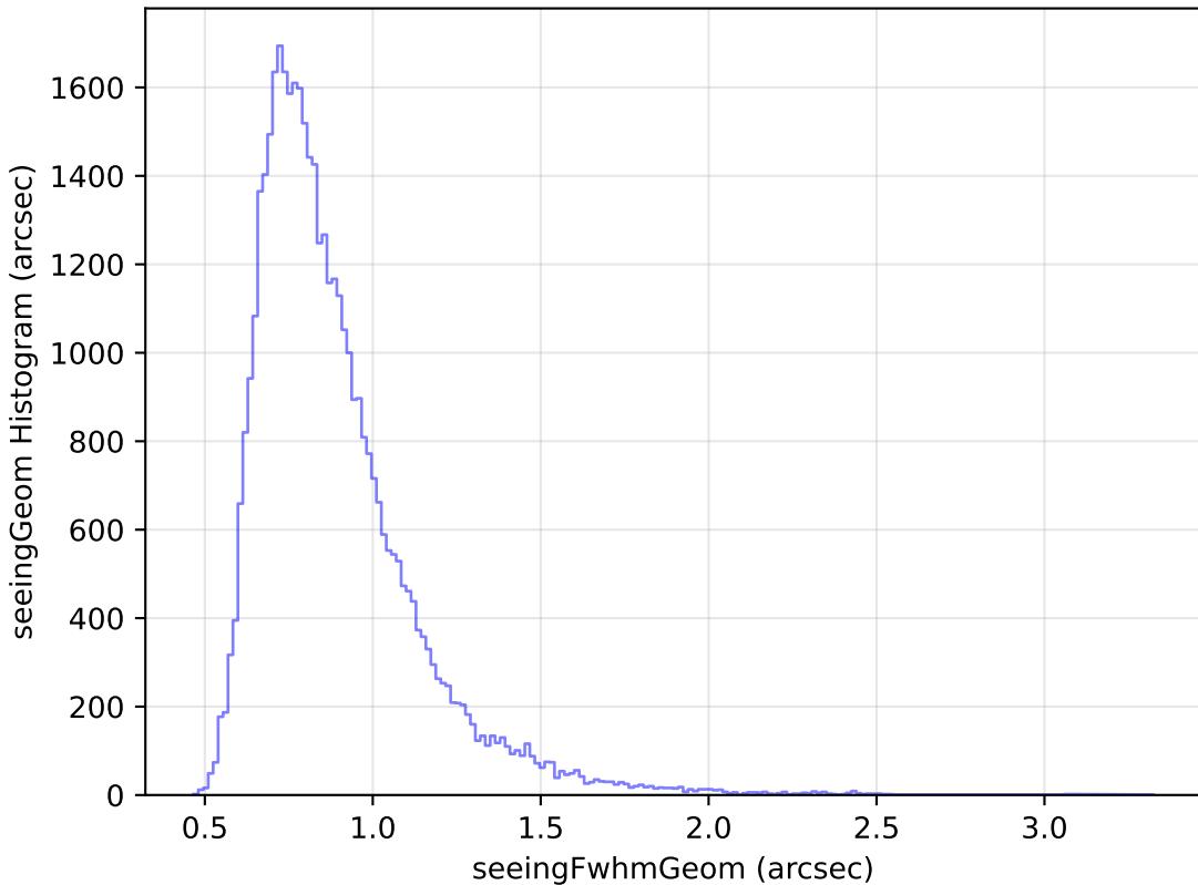
smc_lmc_v3.3_10yrs Yr 1 z band: seeingGeom Histogram
