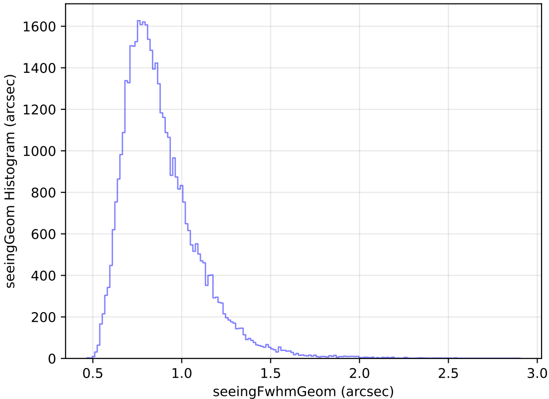
smc_lmc_v3.3_10yrs Yr 1 y band: seeingGeom Histogram
