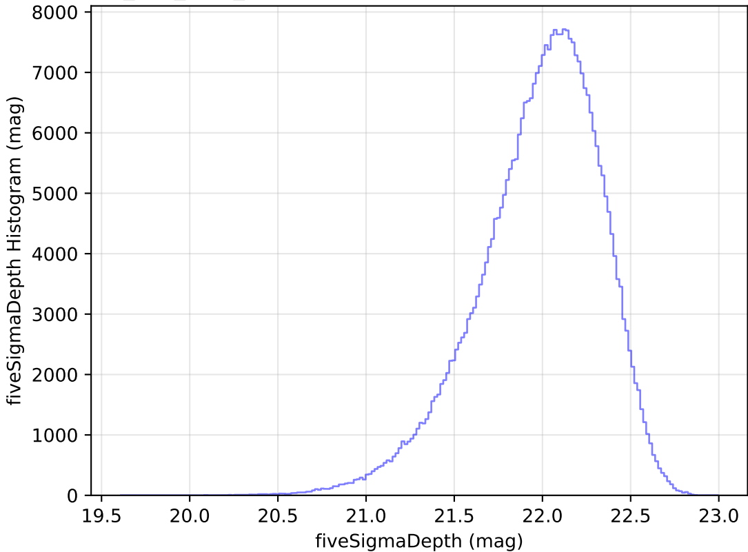
smc_lmc_v3.3_10yrs WFD y band: fiveSigmaDepth Histogram
