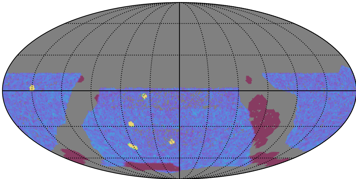
smc_lmc_v3.3_10yrs WFD y band: NVisits
