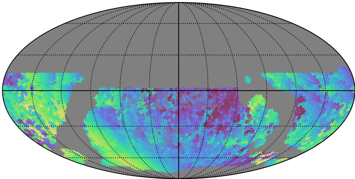
smc_lmc_v3.3_10yrs WFD y band: Min solarElong
