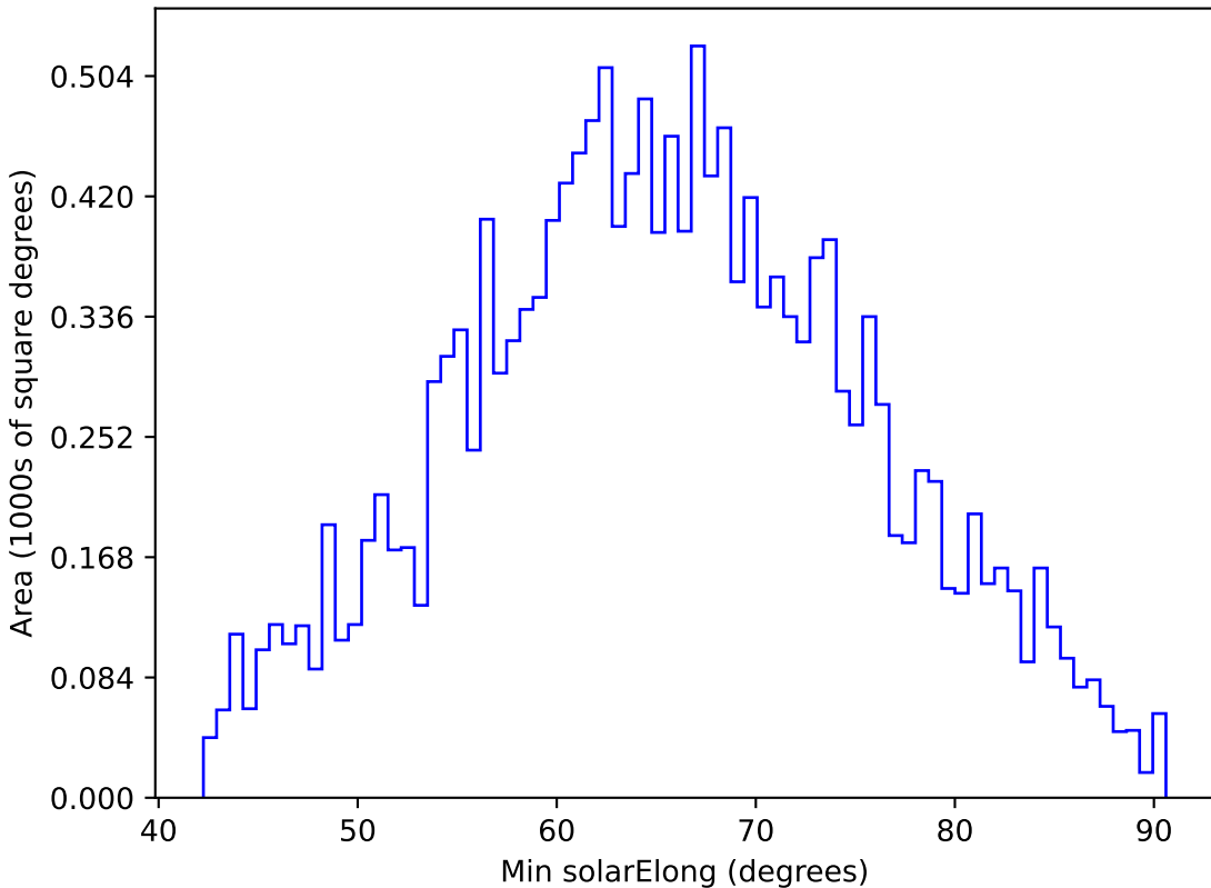
smc_lmc_v3.3_10yrs WFD y band: Min solarElong
