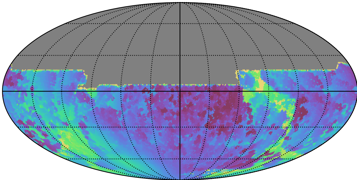
smc_lmc_v3.3_10yrs All sky y band: Min solarElong
