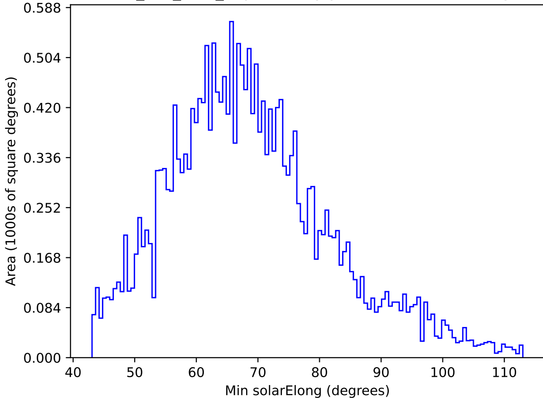
smc_lmc_v3.3_10yrs All sky y band: Min solarElong
