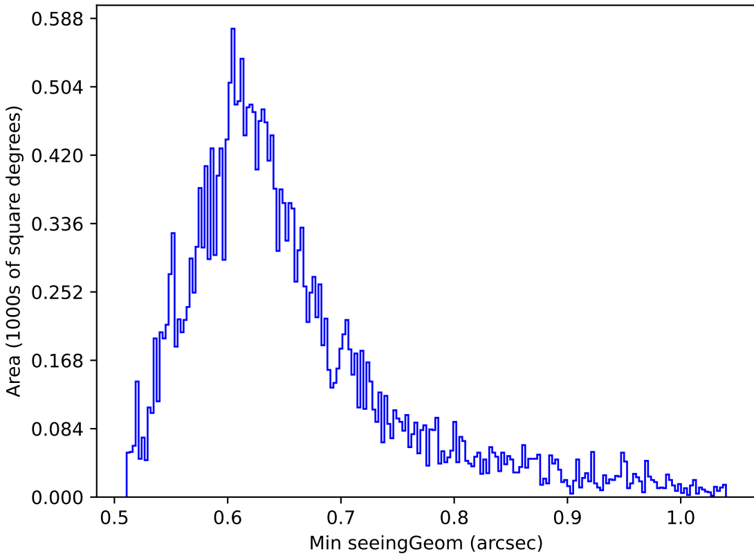
smc_lmc_v3.3_10yrs Yr 1 z band: Min seeingGeom
