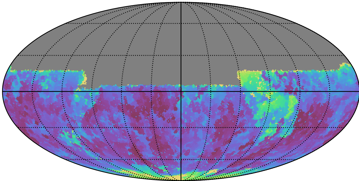
smc_lmc_v3.3_10yrs Yr 1 y band: Min seeingGeom
