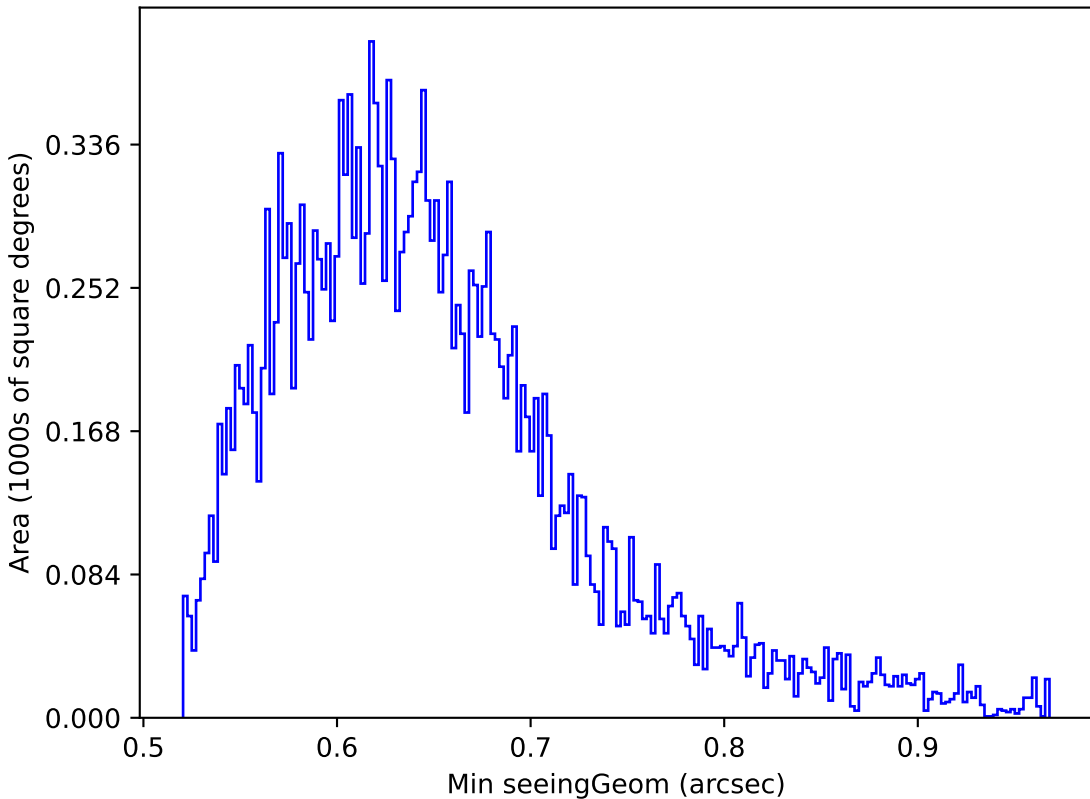
smc_lmc_v3.3_10yrs Yr 1 y band: Min seeingGeom
