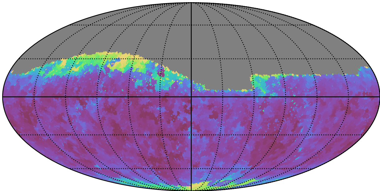
smc_lmc_v3.3_10yrs Yr 1 r band: Min seeingGeom
