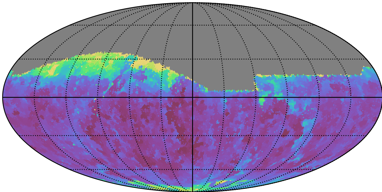
smc_lmc_v3.3_10yrs Yr 1 i band: Min seeingGeom
