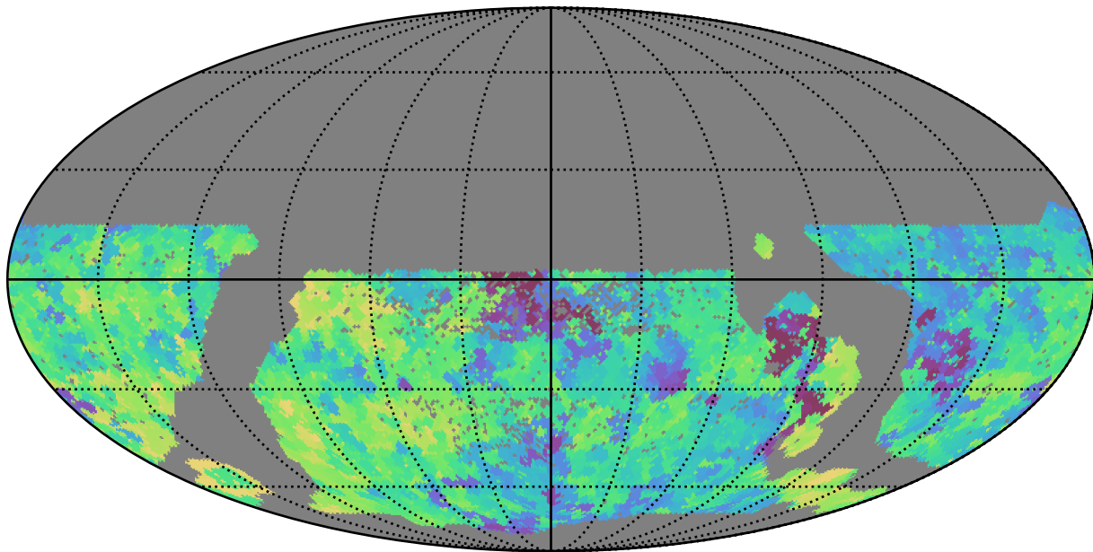
smc_lmc_v3.3_10yrs WFD y band: Min saturation_mag
