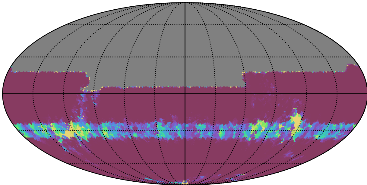
smc_lmc_v3.3_10yrs All sky y band: Min normairmass
