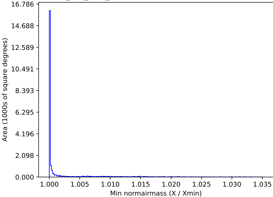
smc_lmc_v3.3_10yrs All sky y band: Min normairmass
