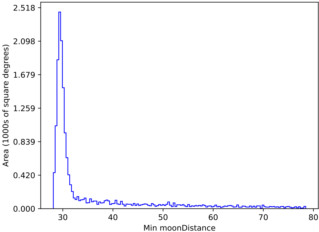
smc_lmc_v3.3_10yrs WFD y band: Min moonDistance
