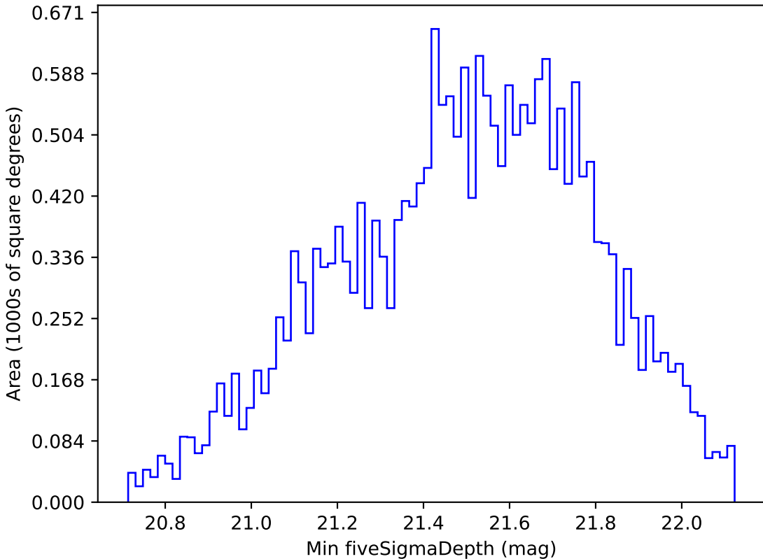
smc_lmc_v3.3_10yrs Yr 1 y band: Min fiveSigmaDepth
