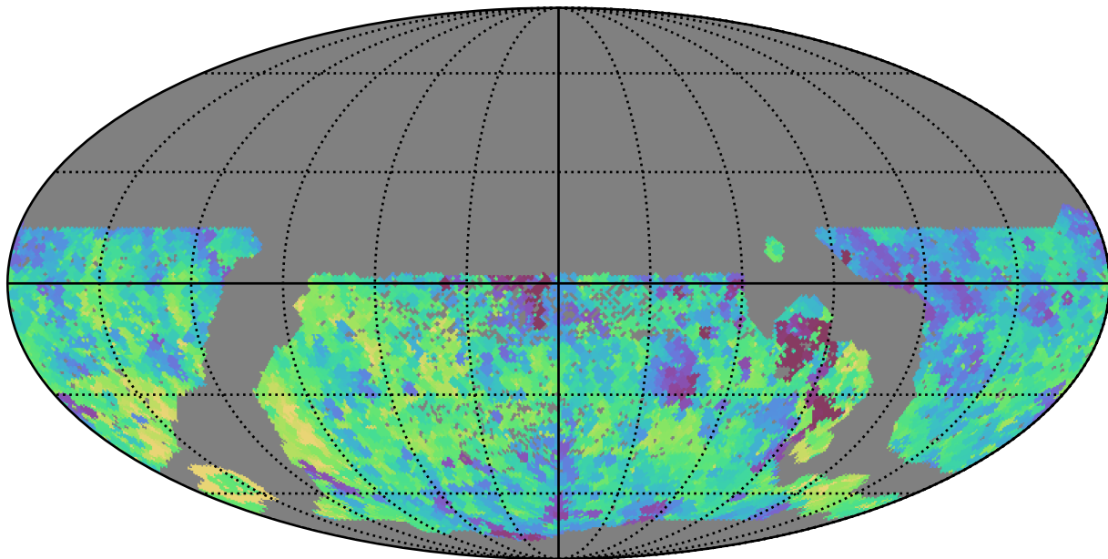
smc_lmc_v3.3_10yrs WFD y band: Min fiveSigmaDepth
