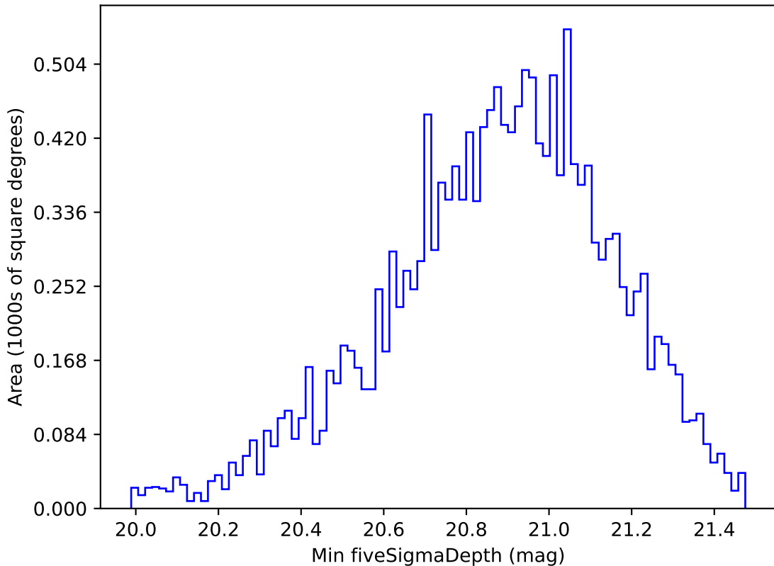
smc_lmc_v3.3_10yrs WFD y band: Min fiveSigmaDepth
