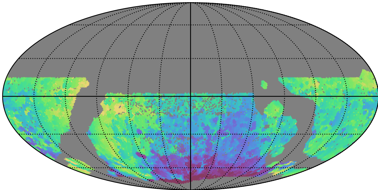
smc_lmc_v3.3_10yrs WFD y band: Min HA
