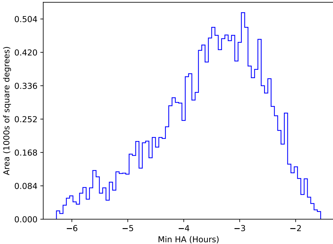
smc_lmc_v3.3_10yrs WFD y band: Min HA
