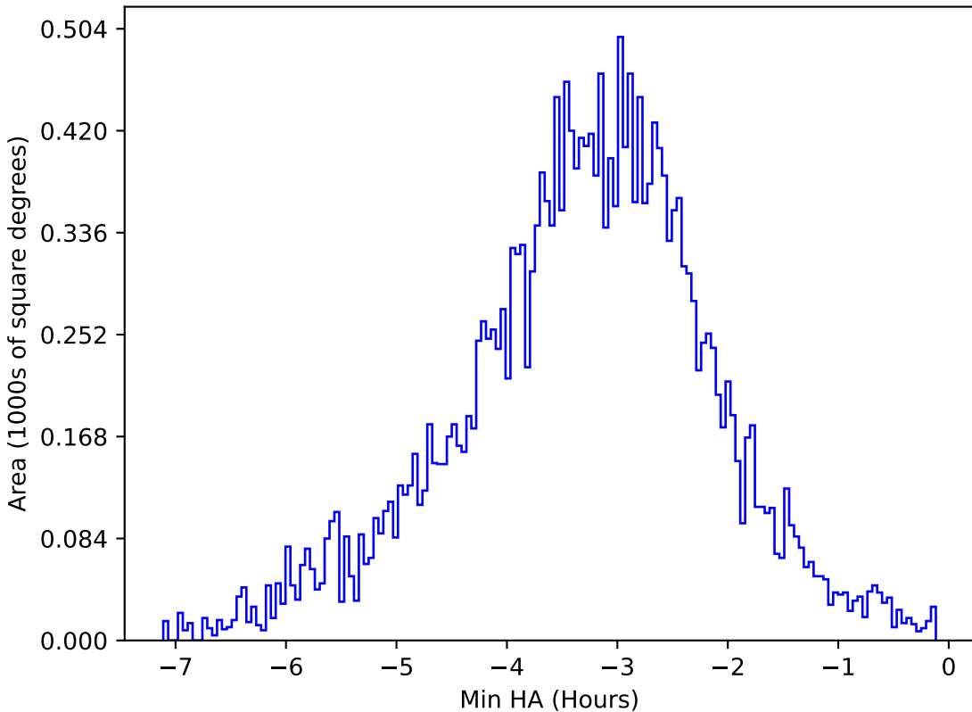
smc_lmc_v3.3_10yrs All sky y band: Min HA
