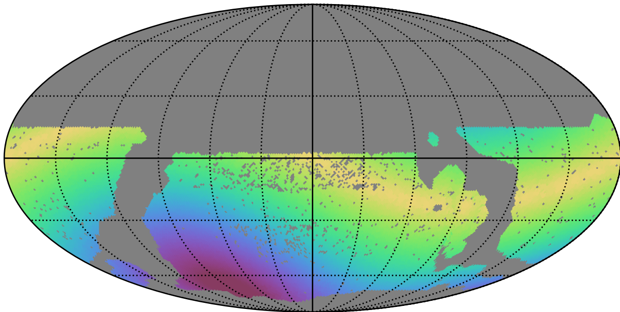
smc_lmc_v3.3_10yrs WFD y band: Max solarElong
