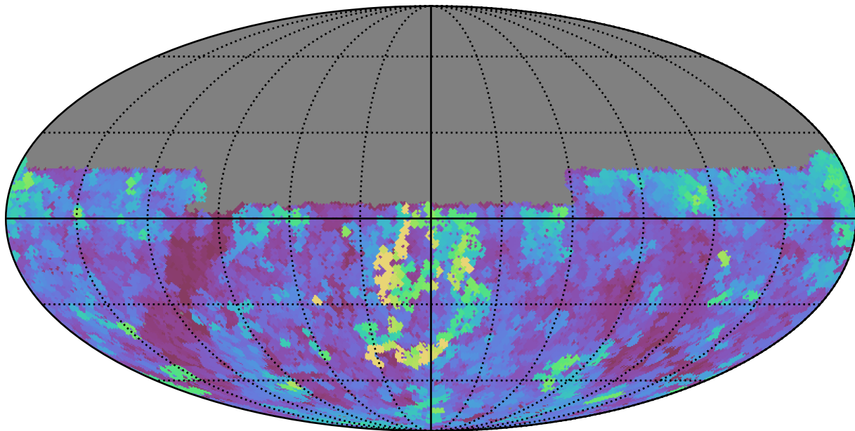
smc_lmc_v3.3_10yrs Yr 1 y band: Max seeingGeom
