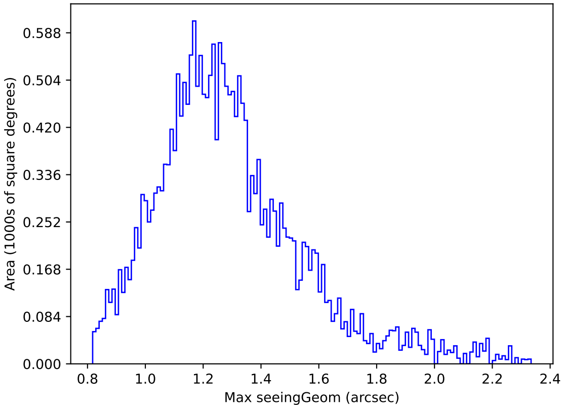
smc_lmc_v3.3_10yrs Yr 1 y band: Max seeingGeom
