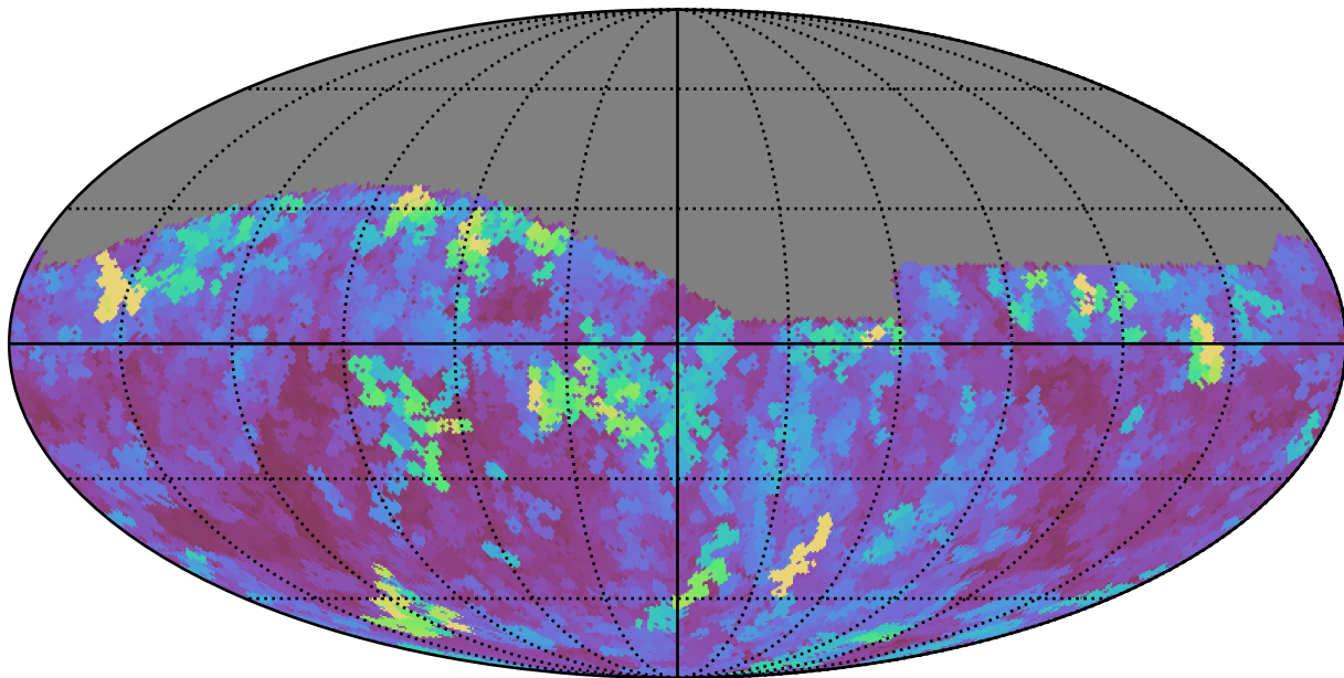
smc_lmc_v3.3_10yrs Yr 1 i band: Max seeingGeom
