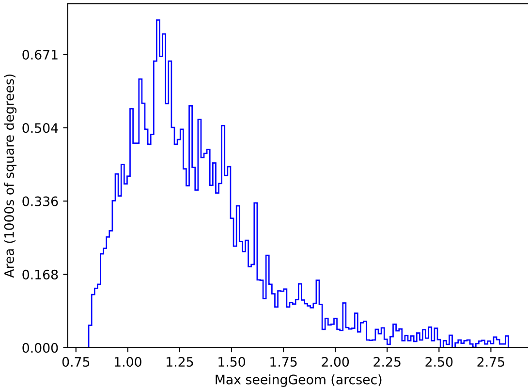
smc_lmc_v3.3_10yrs Yr 1 i band: Max seeingGeom
