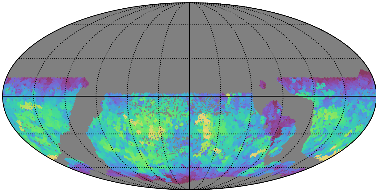
smc_lmc_v3.3_10yrs WFD y band: Max saturation_mag
