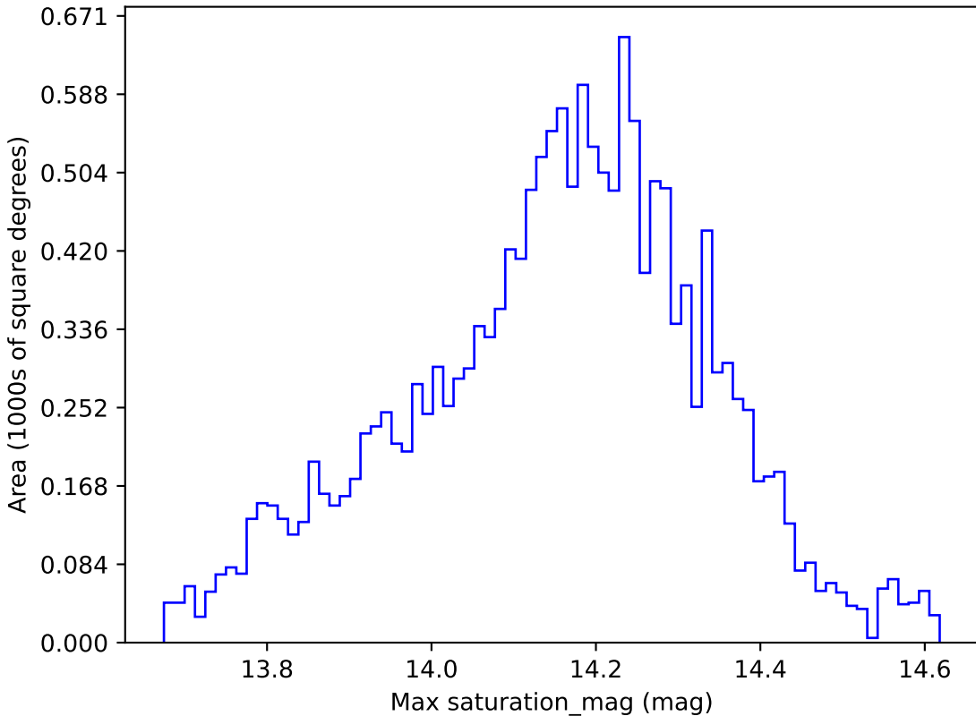
smc_lmc_v3.3_10yrs WFD y band: Max saturation_mag
