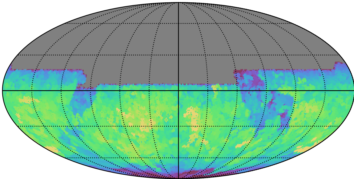
smc_lmc_v3.3_10yrs All sky y band: Max saturation_mag
