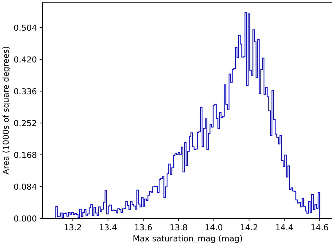
smc_lmc_v3.3_10yrs All sky y band: Max saturation_mag
