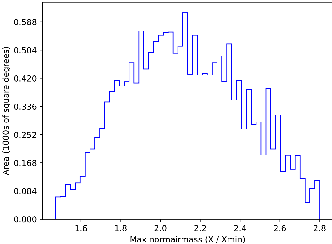
smc_lmc_v3.3_10yrs WFD y band: Max normairmass
