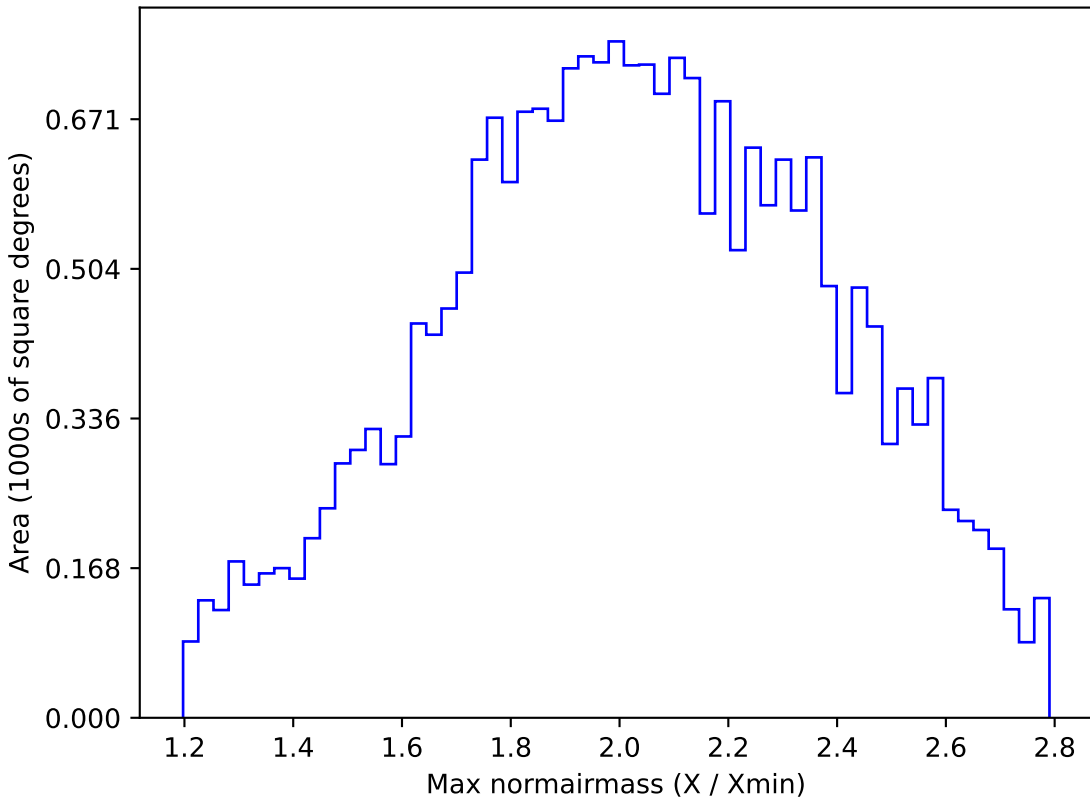
smc_lmc_v3.3_10yrs All sky y band: Max normairmass
