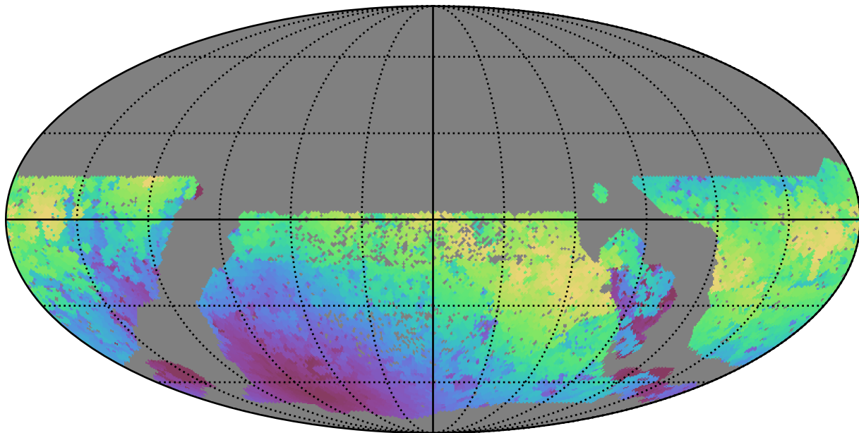
smc_lmc_v3.3_10yrs WFD y band: Max moonDistance
