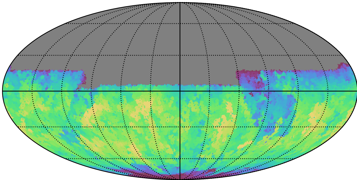
smc_lmc_v3.3_10yrs Yr 1 y band: Max fiveSigmaDepth
