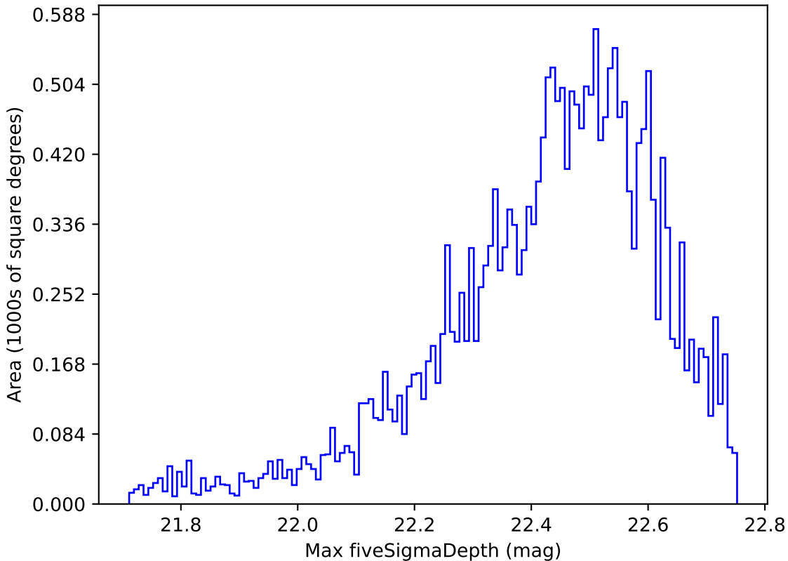
smc_lmc_v3.3_10yrs Yr 1 y band: Max fiveSigmaDepth
