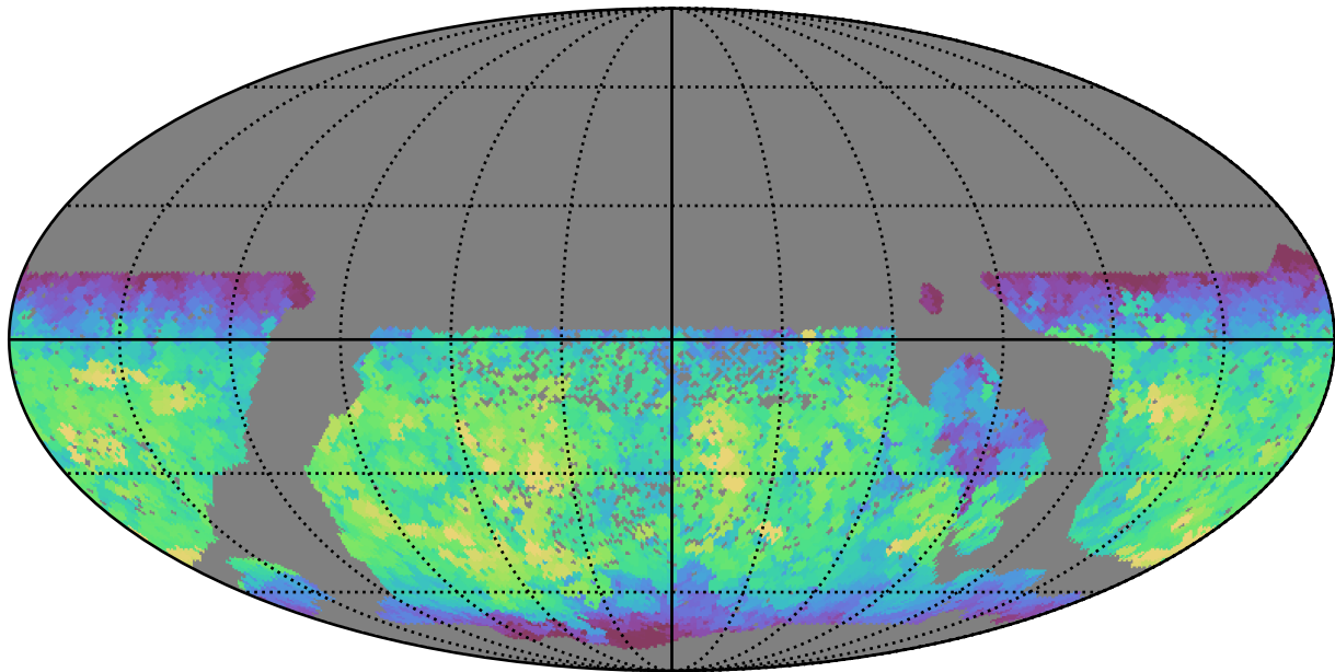
smc_lmc_v3.3_10yrs WFD y band: Max fiveSigmaDepth
