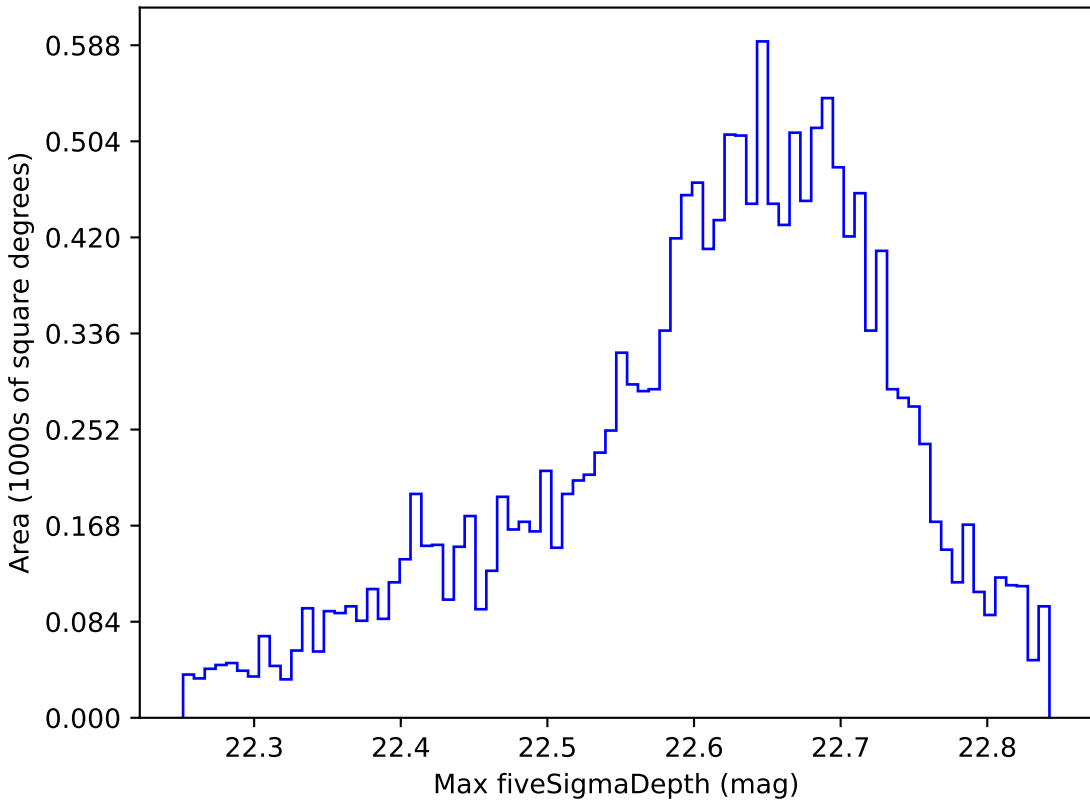
smc_lmc_v3.3_10yrs WFD y band: Max fiveSigmaDepth
