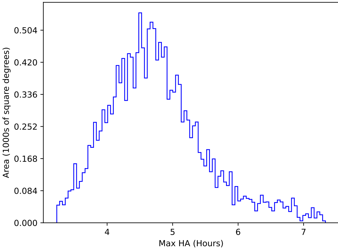
smc_lmc_v3.3_10yrs WFD y band: Max HA
