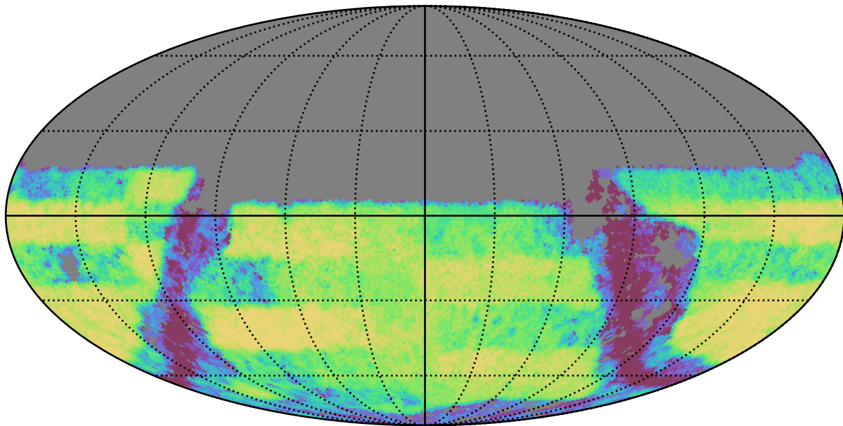
smc_lmc_v3.3_10yrs Yr 3-4 y band: Exgal_CoaddM5
