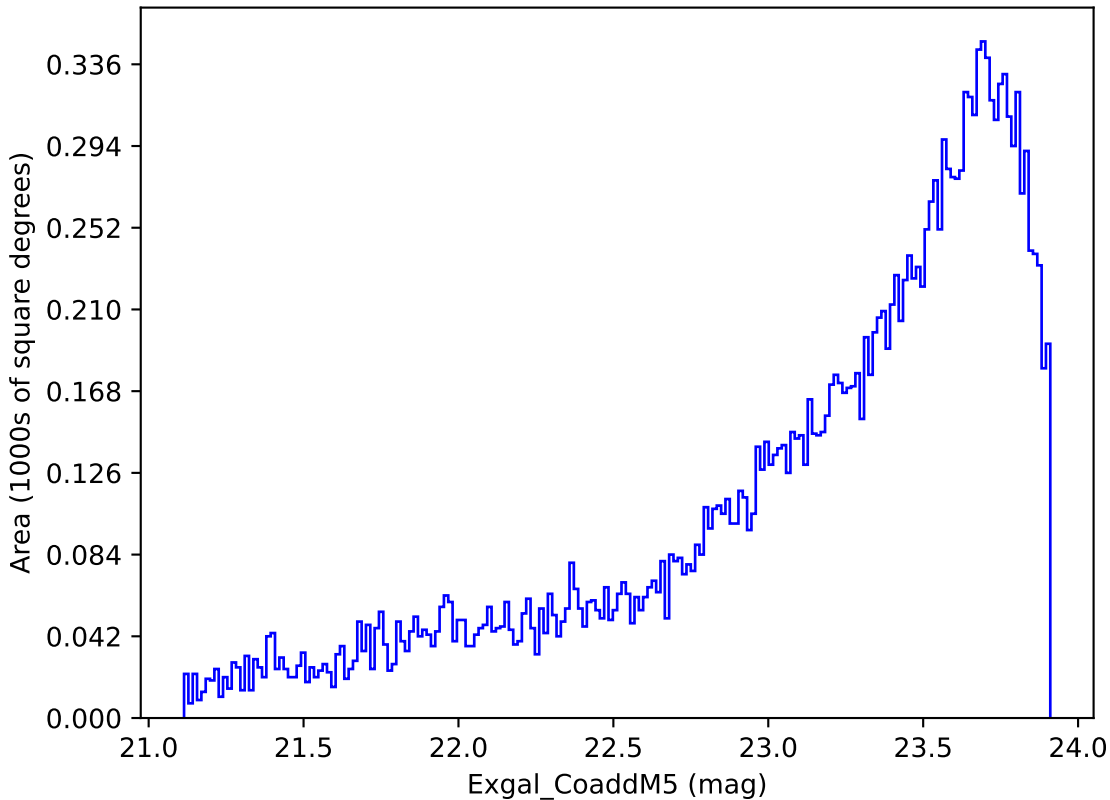
smc_lmc_v3.3_10yrs Yr 3-4 y band: Exgal_CoaddM5
