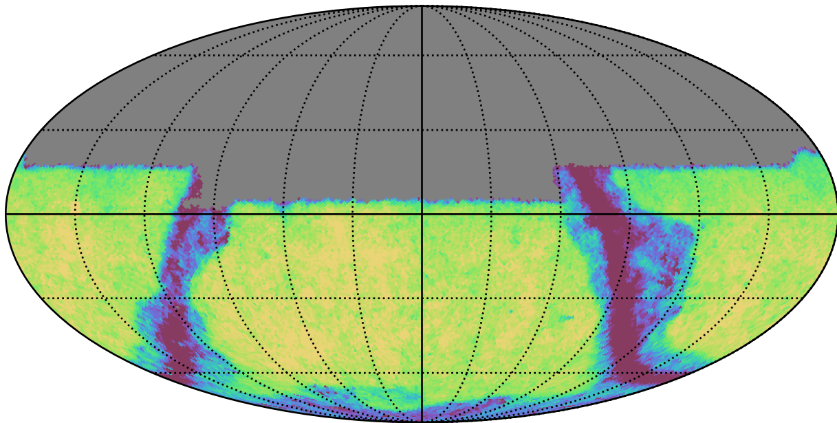
smc_lmc_v3.3_10yrs Yr 1 y band: Exgal_CoaddM5
