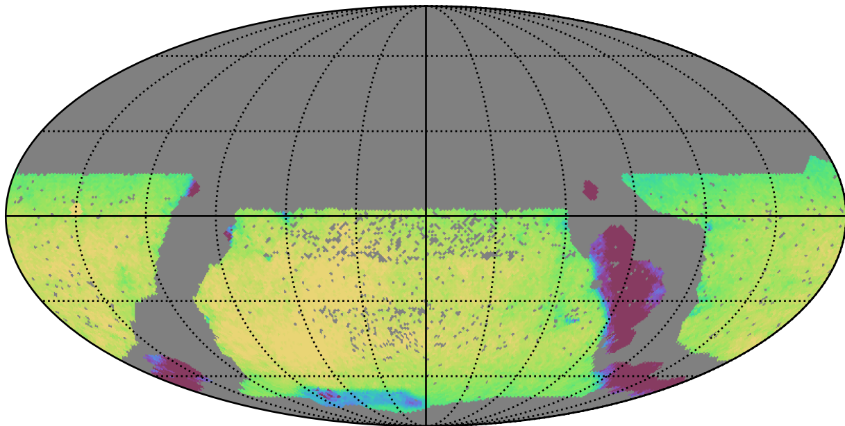
smc_lmc_v3.3_10yrs WFD y band: Exgal_CoaddM5
