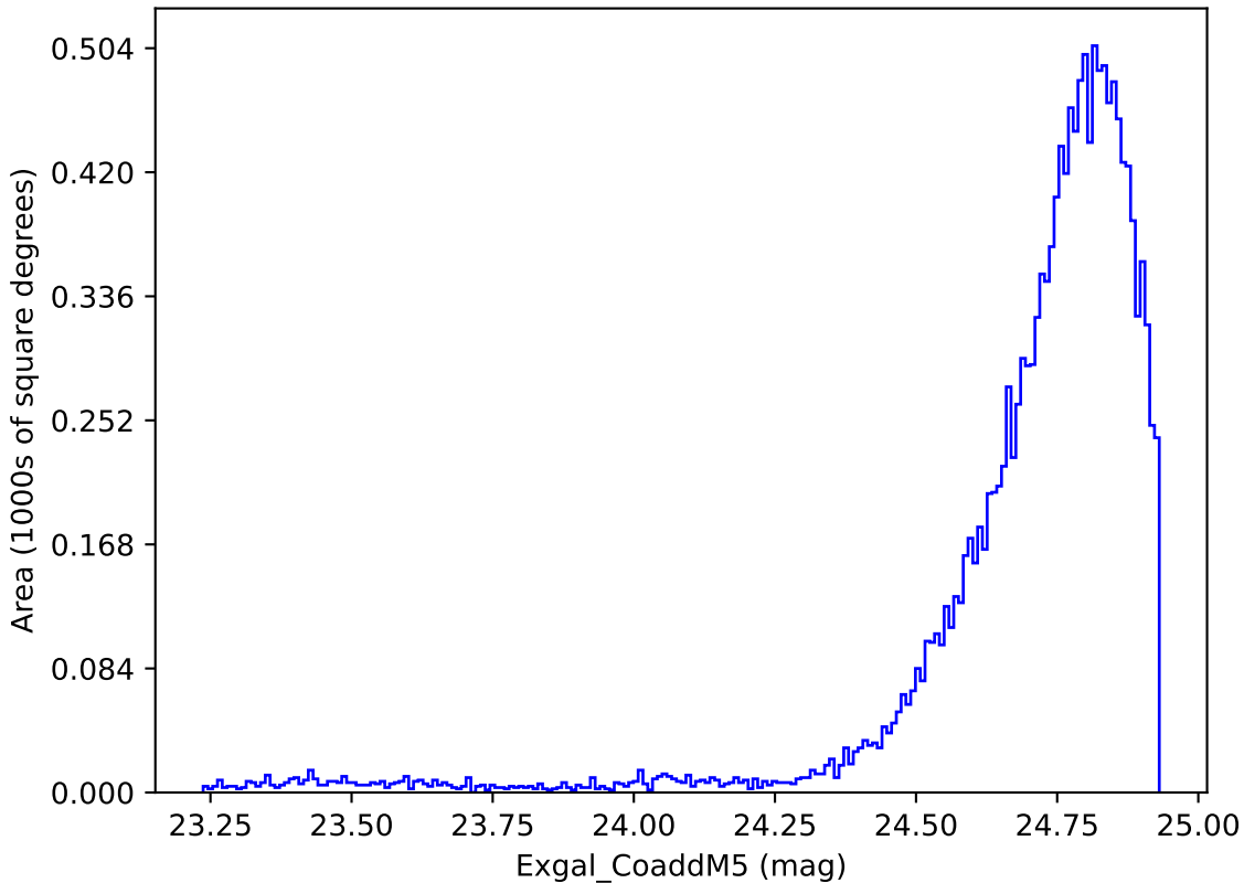
smc_lmc_v3.3_10yrs WFD y band: Exgal_CoaddM5
